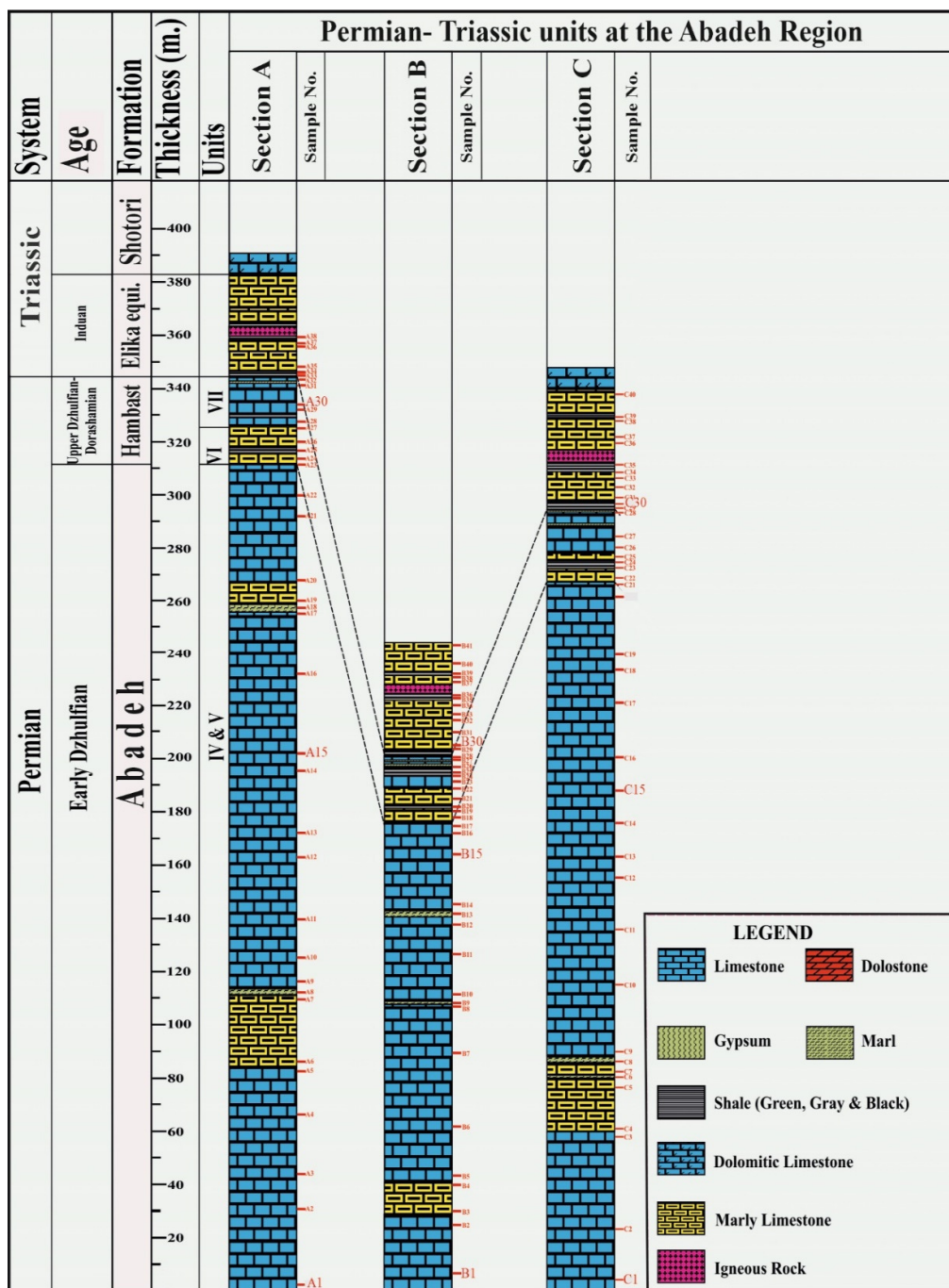
شکل ۳. ستون‌های چینه‌شناسی برش‌های مورد مطالعه در ناحیه آبادیه Fig. 3. Stratigraphic column of studied sections at the Abadeh area
