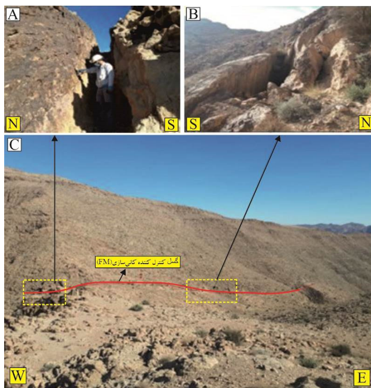
شکل ۱۰. تصویر موقعیت گسل (FM)، کنترل‌کننده کانی‌سازی، کانسار پیرحاجات. A: قسمتی از گسل اصلی در غرب محدوده، B: قسمتی
