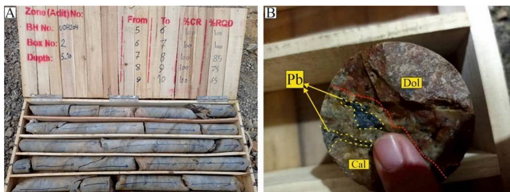
شکل ۲۲. A: مغزه‌های مربوط به یک جعبه حفاری، B: کانی‌سازی سرب در مغزه‌های حاصل از حفاری، گمانه UDH204، کانسار پیرحاجات، طیس.
