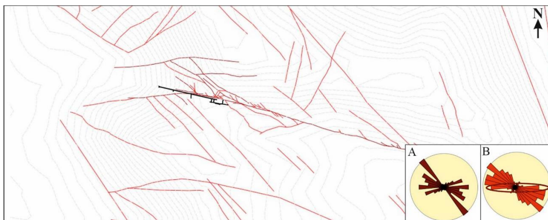
شکل ۱۱. نقشه گسل‌های برداشت شده به همراه رزداگرام، A: رزداگرام روند ماده معدنی، B: رزداگرام گسل‌های محدوده، با تغییرات اندک از اسدی (۱۴۰۰). کانسار پیرحاجات.
