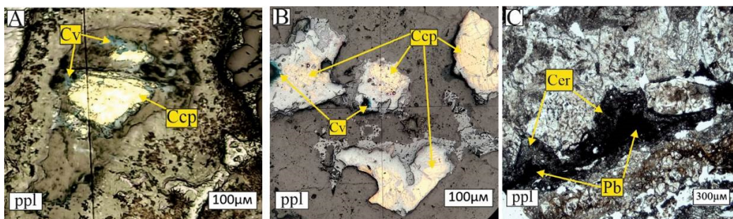
شکل ۱۴. A و B: جانشینی کانی کالکوپیریت و کوولیت، C: جانشینی کانی سرب طبیعی و سروزیت، کنسار پیرحاجات. Ccp: کالکوپیریت، Cv: کوولیت، pb: سرب طبیعی، Cer: سروزیت. (حروف اختصاری کانی‌ها از ویتنی و ایوانز، ۲۰۱۰).
