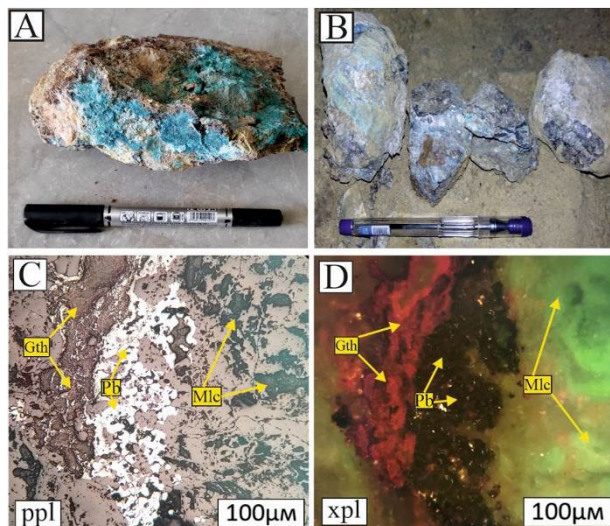
شکل ۱۵. A: نمونه دستی از کانی مالاکیت، آزوریت و کریزوکلا، B: نمونه دستی از کانی سازی آزوریت همراه با سرب طبیعی در زمینه سیلیسی، C و D: تصویر میکروسکوپی از مالاکیت، سرب طبیعی و گوئیت، کنسار پیرحاجات. Pb: سرب طبیعی، Gth: گوئیت، Mlc: مالاکیت. PPL: نور طبیعی، XPL: نور پلاریزه. (حروف اختصاری کانی‌ها از ویتنی و ایوانز، ۲۰۱۰)
