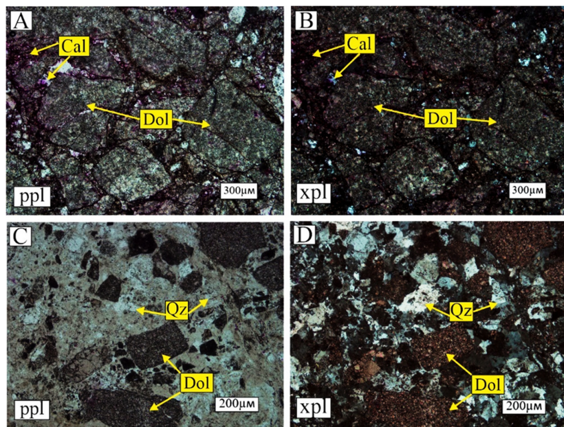
شکل ۶. A و B: تصویر میکروسکوپی سنگ میزبان برشی شده (تراز ۱۲۰۵ متر)، C و D: تصویر میکروسکوپی کانسنگ برشی با سیمان کوارتز و کلسیت (تراز ۱۲۲۵ متر)، کانسار پیرحاجات. Dol: دولومیت، Cal: کلسیت، Qz: کوارتز. PPL: نور عبوری عادی، XPL: نور عبوری متقاطع (حروف اختصاری از ویتنی و ایوانز، ۲۰۱۰)
