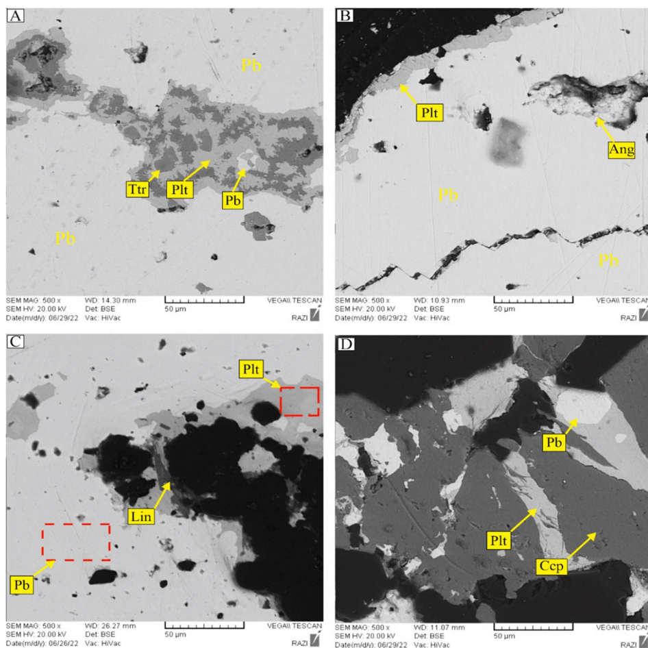
شکل ۱۷. تصاویر میکروسکوپ الکترونی (BS) از نمونه PT.30.123، Zone 1: A، کانی‌های تتراهدریت (Ttr) و پلاتنریت (Plt) و سرب طبیعی (Pb) که به صورت زمینه است، Zone 2: B، کانی‌های پلاتنریت (Plt) و آنگلزیت (Ang) و سرب طبیعی (Pb)، Zone 3: C، کانی‌های لیناریت (Lin)، پلاتنریت (Plt) و سرب طبیعی (Pb)، Zone 4: D، کانی‌های پلاتنریت (Plt)، کالکوپریت (Ccp) و سرب طبیعی (Pb)، کانسار پیرحاجات. (حروف اختصاری کانی‌ها از ویتنی و ایوانز، ۲۰۱۰)
