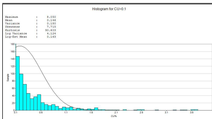
شکل ۴. توزیع تجمعی عیارهای بالای ۰/۱ درصد نمونه‌های کانسار تکنار
