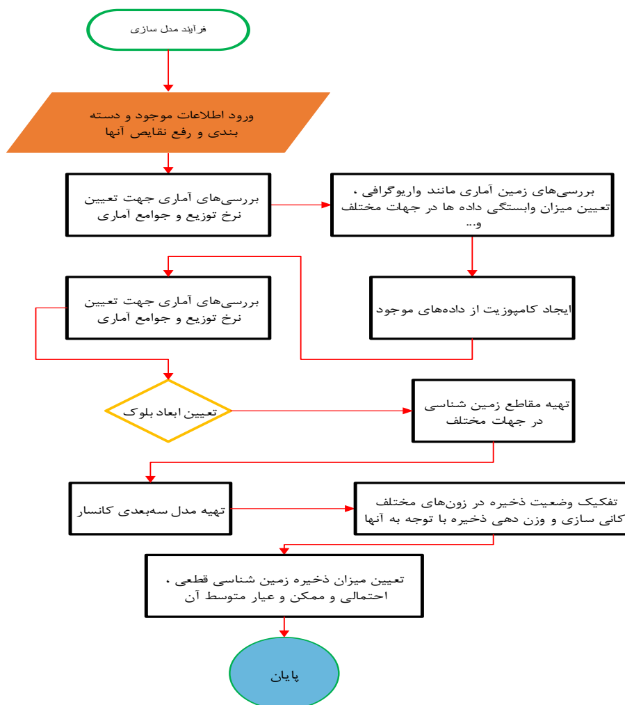
شکل ۱. فرآیند کلی مدل‌سازی نرم‌افزاری ذخایر معدنی (حمداد، ۱۳۹۶)
