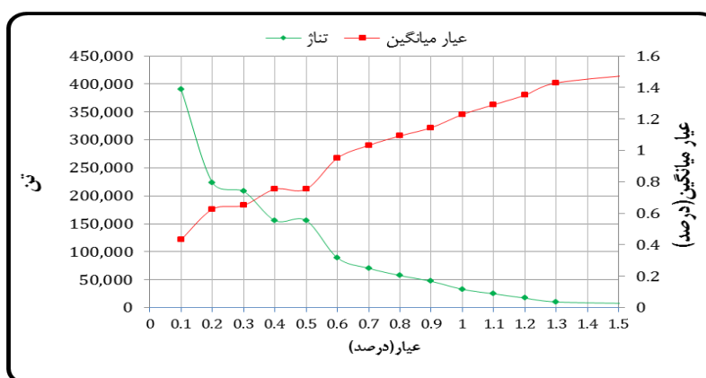
شکل ۱۱. نمودار عیار-تناژ مدل حاصل از تخمین کریجینگ معمولی کانسار تکنار
